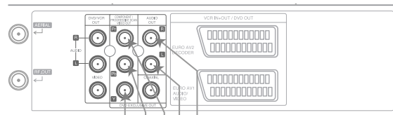
Rückseite dieses Geräts (Anschluss des DVD-Ausgangs)
