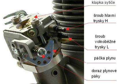
Walbro WT 561
