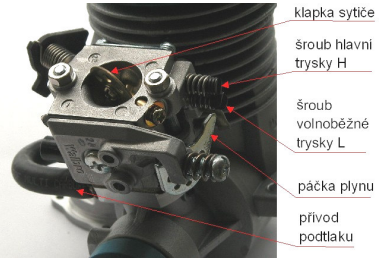
Walbro WT 481
