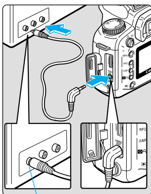
Borne d'entrée vidéo
