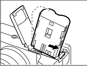
Cierre de la batería
