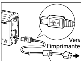
Prise DIGITAL (Numérique) Câble de liaison directe DIF-100
