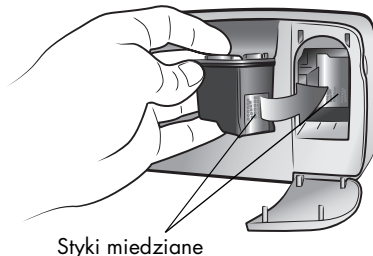
Styki miedziane
