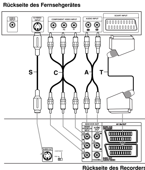
Rückseite des Recorders
