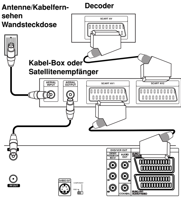
Rückseite des Recorders
