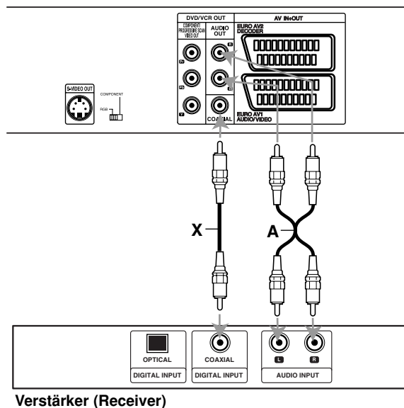
Rückseite des Recorders
