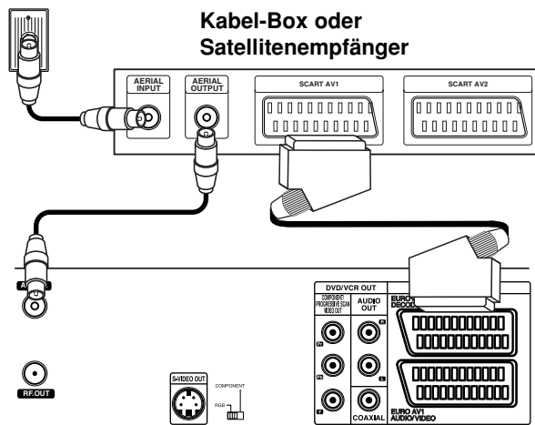
Rückseite des Recorders
