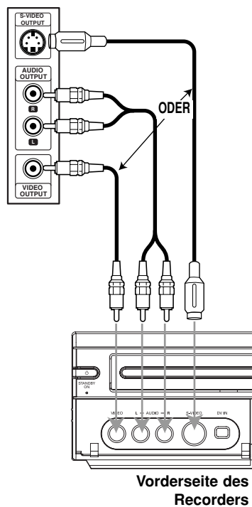
Anschlussleiste einer Zubehörkomponente (VCR, Comcorder, etc.)
